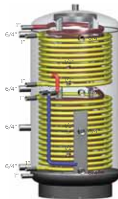
Systemspeicher WR mit Edelstahlwellrohr-Wärmetauscher und 2 Solarregister
