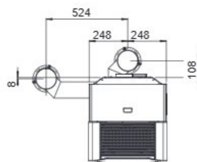
BOVENAANZICHT
