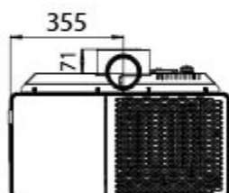
BOVENAANZICHT
