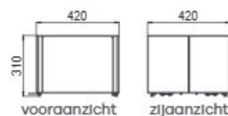
vooraanzicht
