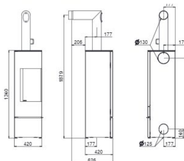
CONNECT WOOD zonder accumulatiemassa
