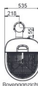
Bovenaanzicht
