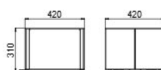
Vooraanzicht Zij aanzicht
