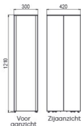
KAST Breedte 300 mm
