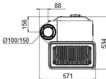
Bovenaanzicht PGI
