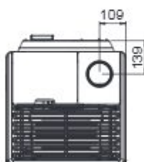
Bovenaanzicht RAO
