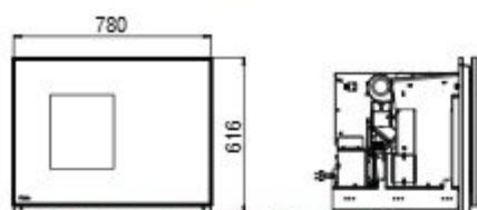
E15554 standaardkader, smal
