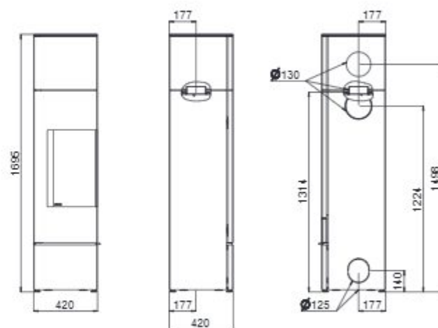
CONNECT WOOD met accumulatiemassa
