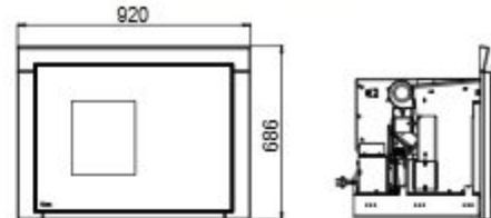
E15810 groot kader met spoiler
