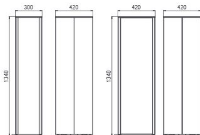
Vooraanzicht Zij aanzicht
