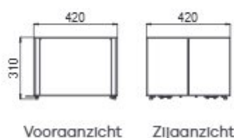
BANK Breedte 420 mm
