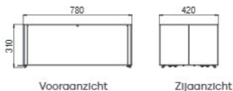
BANK Breedte 780 mm
