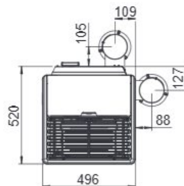
Bovenaanzicht
