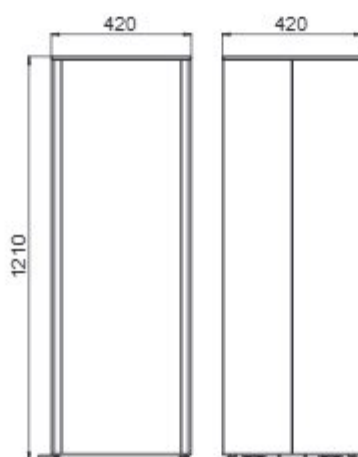
Vooraanzicht
