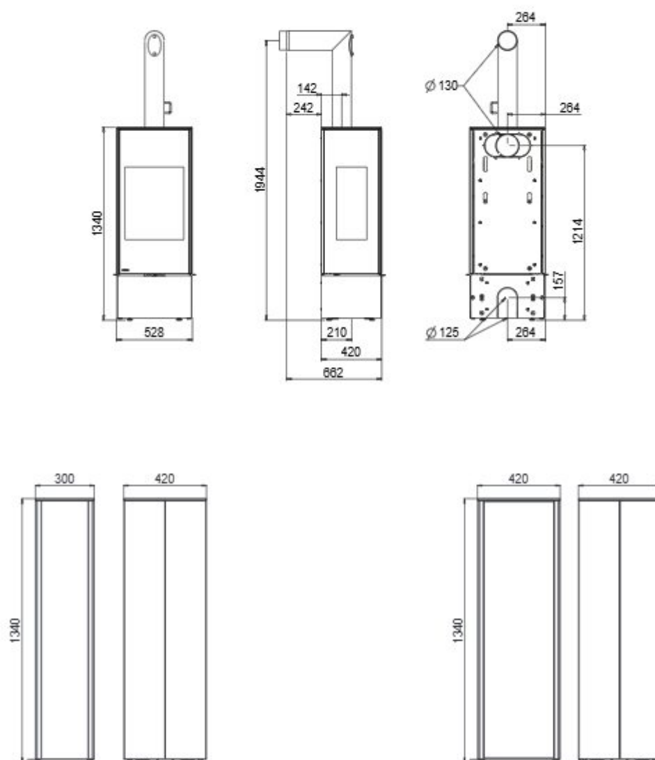
Vooraanzicht Zij aanzicht
