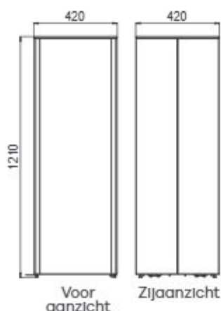
KAST Breedte 420 mm
