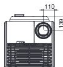
Bovenaanzicht PGI
